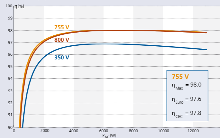
Wirkungsgradkennlinien Powador 14.0 TL3
